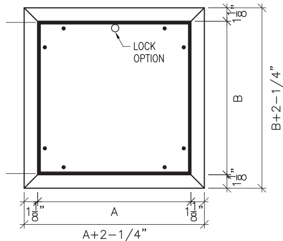
Elevation
